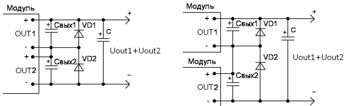
Рисунок 5.6 - Примеры последовательного соединения выходных каналов модулей для получения повышенного выходного напряжения.
